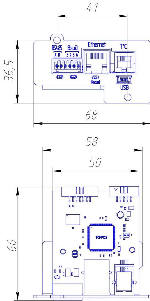
Рисунок 1.2 – Габаритные размеры изделия
